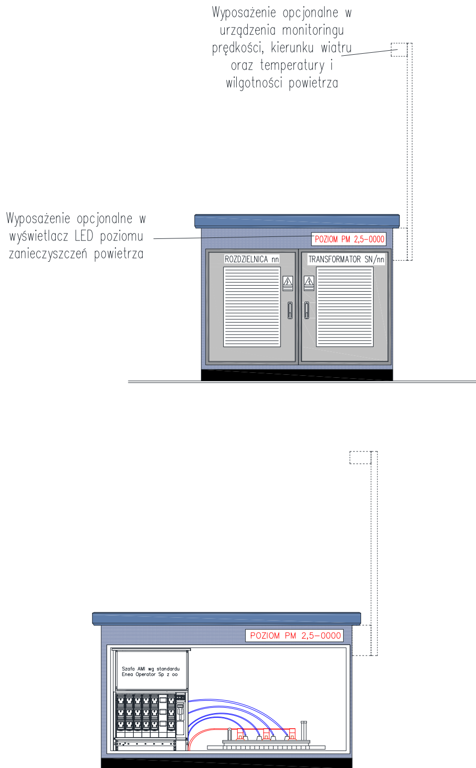
Rysunek nr 7. Wyposażenie opcjonalne stacji transformatorowej kompaktowej prefabrykowanej SN/nn
