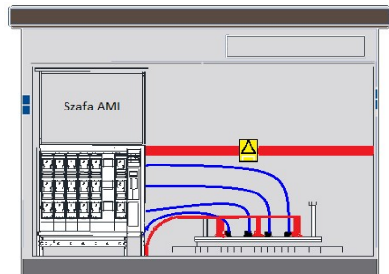
Rysunek nr 5. Widok wnętrza stacji
