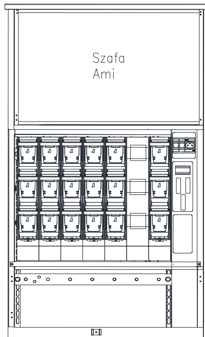
Rysunek nr 2. Rozmieszczenie elementów w rozdzielni nn (dopuszcza się wykonanie lustrzane)
