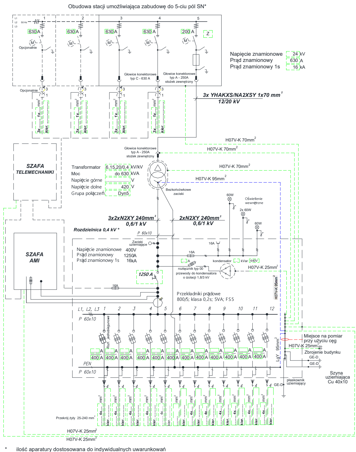
Rysunek nr 1. Schemat ideowy stacji SN/nn do 630 kVA
