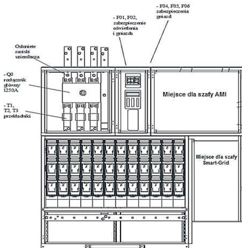
Rysunek nr 2. Rozmieszczenie elementów w rozdzielni nn (dopuszcza się wykonanie lustrzane)
