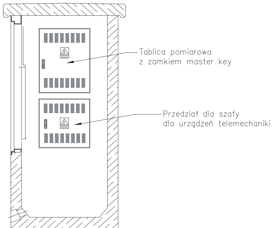
Rysunek nr 4d. Widok umieszczenia drzwi do liczników układu pomiarowego urządzeń w złączu kablowym SN –z układem pomiarowo rozliczeniowym (dopuszcza się lustrzane odbicie).
