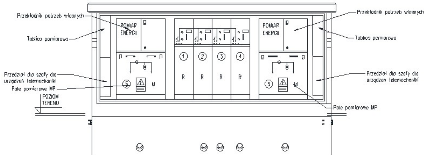
Rysunek nr 4i. Widok rozmieszczenia urządzeń w złączu pomiarowym SN z dwoma układami pomiarowo-rozliczeniowymi pośrednimi
