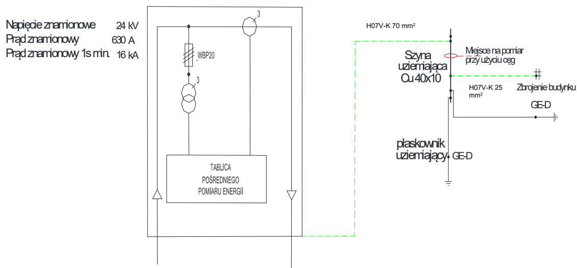
Rysunek nr 4h. Schemat złącza pomiarowego SN z układem pomiarowo-rozliczeniowym pośrednim
