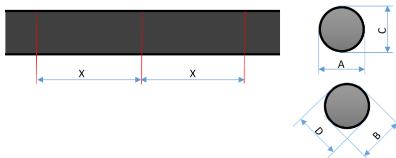
Rys. 6. Pomiar średnicy zewnętrznej kabla. Oznaczenie miejsc pomiarowych
