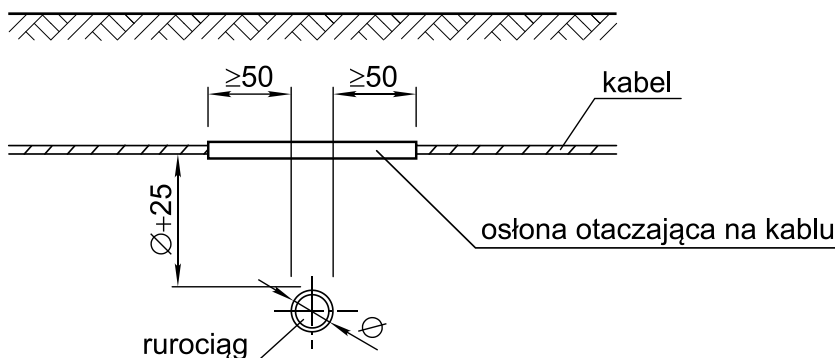
Rys. 5.17 Przekrój skrzyżowania rurociągu wodociągowego, ściekowego, ciepłego lub gazowego z gazem niepalnym z kablem elektroenergetycznym o napięciu U_N \leq 30 \text{ kV} (wymiar w cm)
