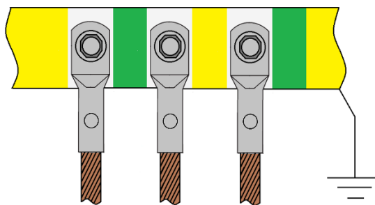
Rys. 3. Sposób przyłączenia żył powrotnych kabla do instalacji uziemiającej
