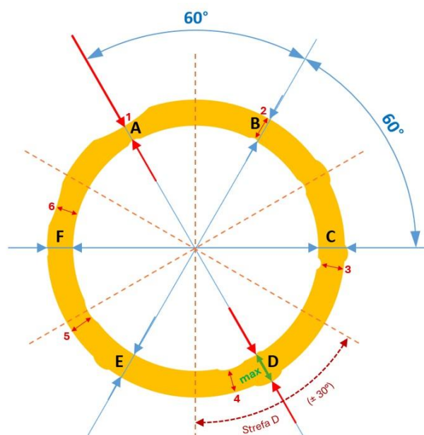
Rys. 4. Metodologia pomiaru grubości izolacji zgodnie z [18, 19, 30]
