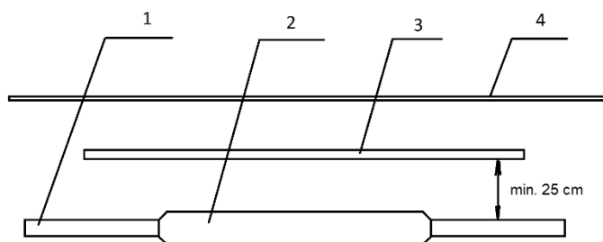
Rys. 5.10 Ochrona mufy przed uszkodzeniami mechanicznymi w gruntach wymagających zagęszczenia mechanicznego 1 – kabel, 2 – mufa, 3 – płyta ochronna, 4 – taśma ostrzegawcza
