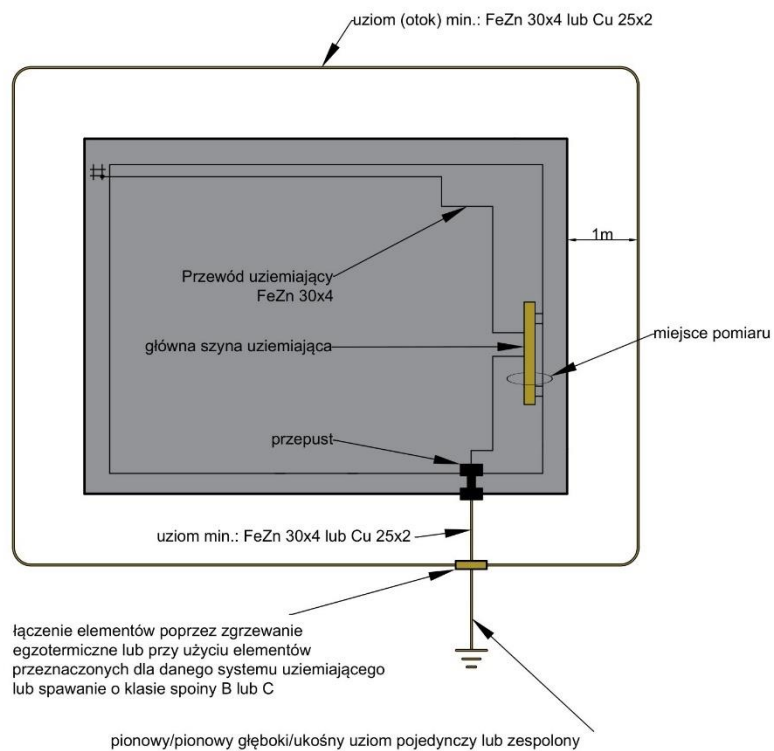
Rys. 4. Kompaktowa stacja transformatorowa, szafa/złącze kablowe SN na terenie ZIU - rzut.
