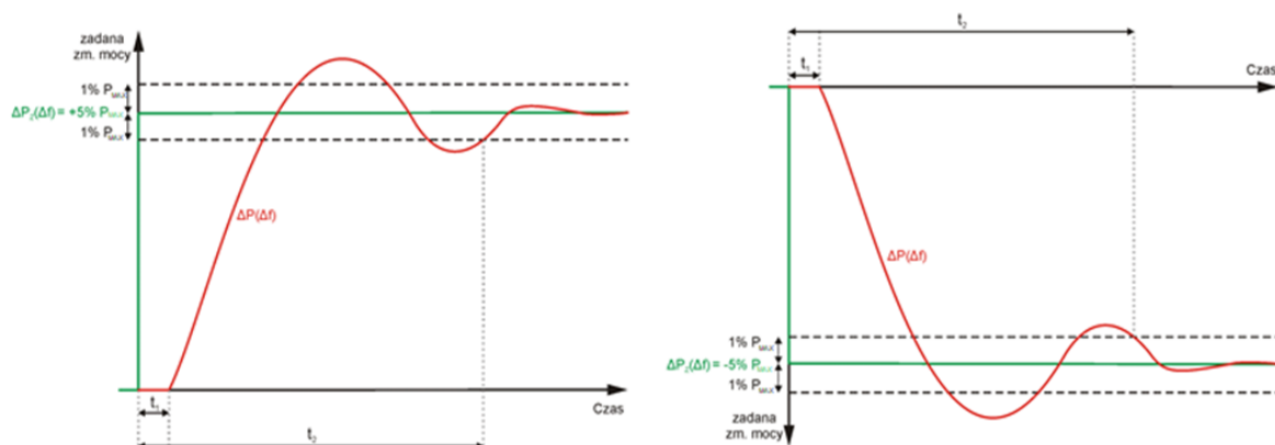
Rys. 2 Kryterialne czasy oceny odpowiedzi częstotliwościowej.
