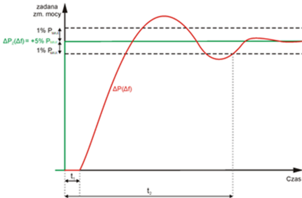
Rys. 3 Kryterialne czasy oceny odpowiedzi częstotliwościowej.
