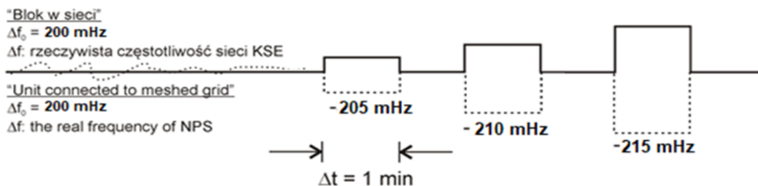
Rys. 1 Sprawdzenie niewrażliwości odpowiedzi częstotliwościowej.
